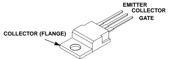
JEDEC TO-220AB
