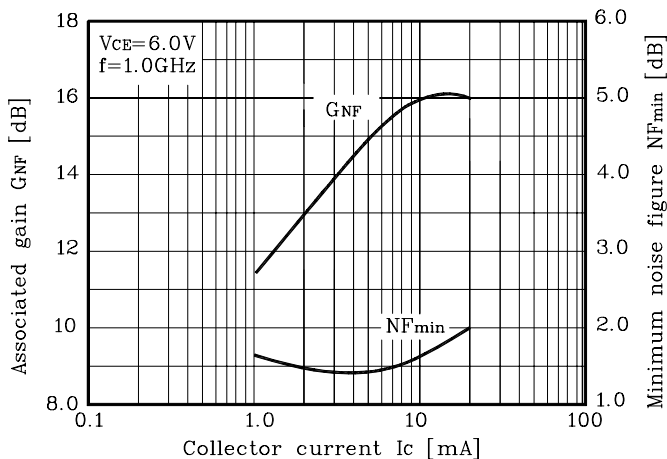
Fig. 17 NF min ,G NF -I c
