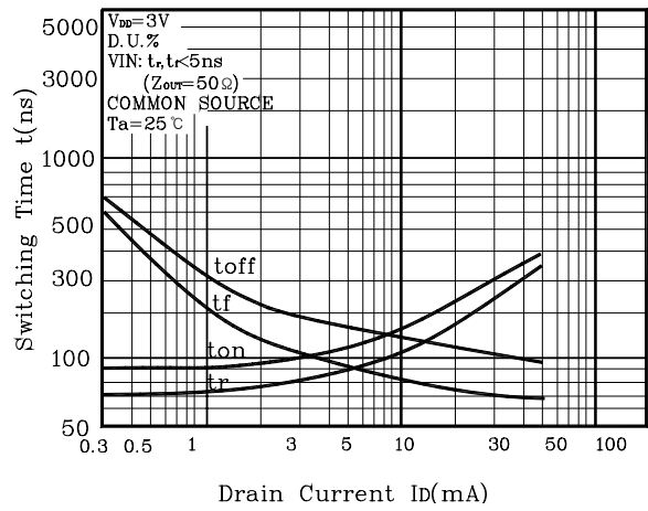
Fig.8 t - I_D
