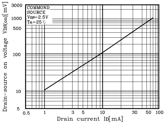
Fig.7 V_{DS} - I_D
