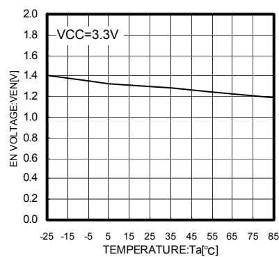
Fig.10 Ta-Icc
