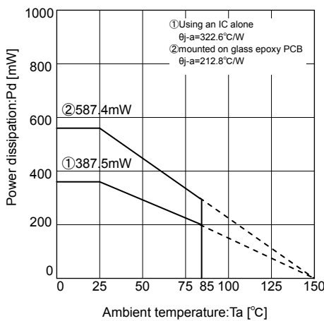
Fig.26 Thermal derating curve (MSOP8)
