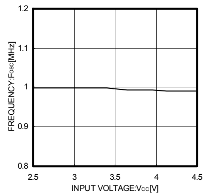
Fig.11 Vcc-Fosc
