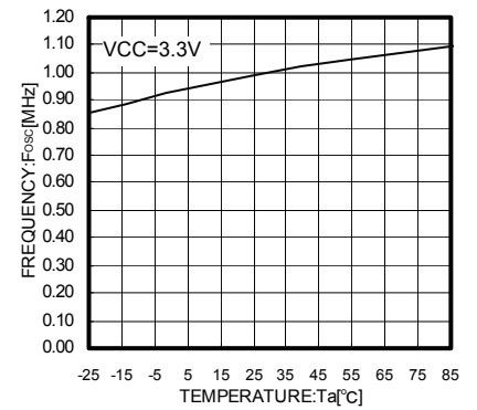
Fig.8 Ta - Fosc
