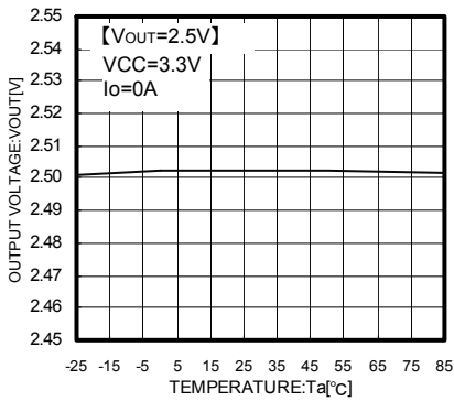
Fig.6 Ta-Vout
