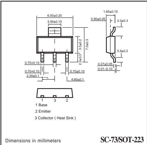
SC-73/SOT-223
