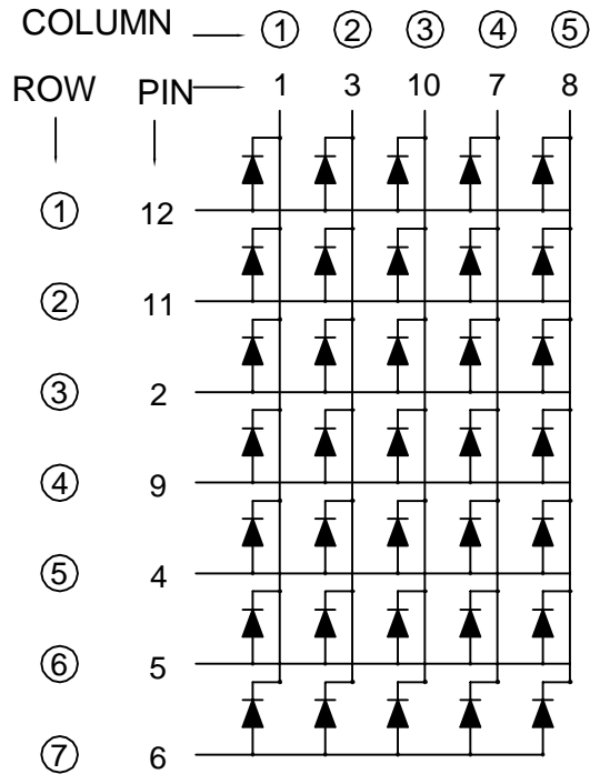
LMD5701ASR-XX-PF
