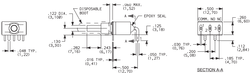
E121SD1AGE SPDT
