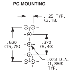
E121SD3_GE SPDT
