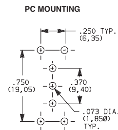
E121SD3V_GE SPDT
