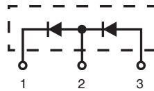
ISOPLUS 220 E153432
