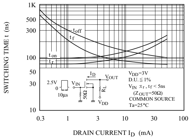
t - I_D
