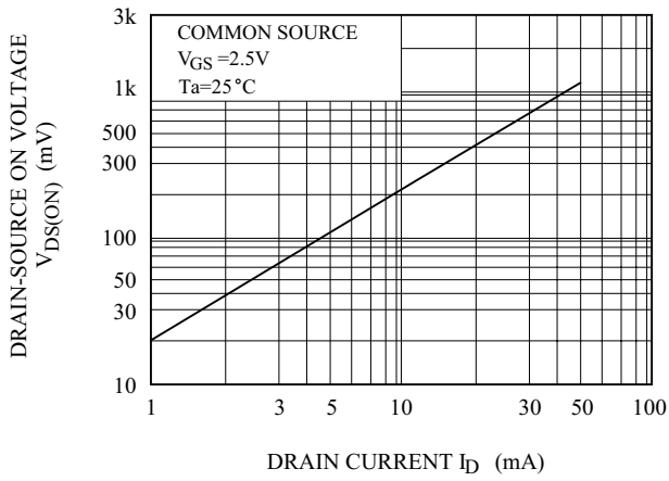
V_{DS(ON)} - I_D
