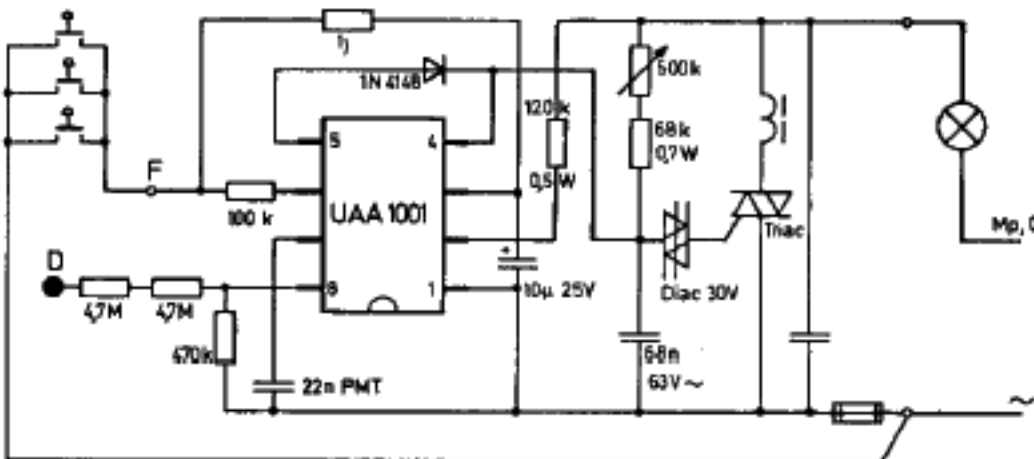
Bild 1: Anwendungsschaltung für den UAA 1001
