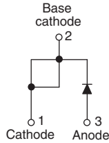
VS-15ETL06PbF
