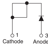
VS-15ETL06FPPbF
