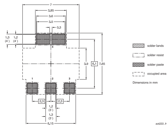
SOT223
