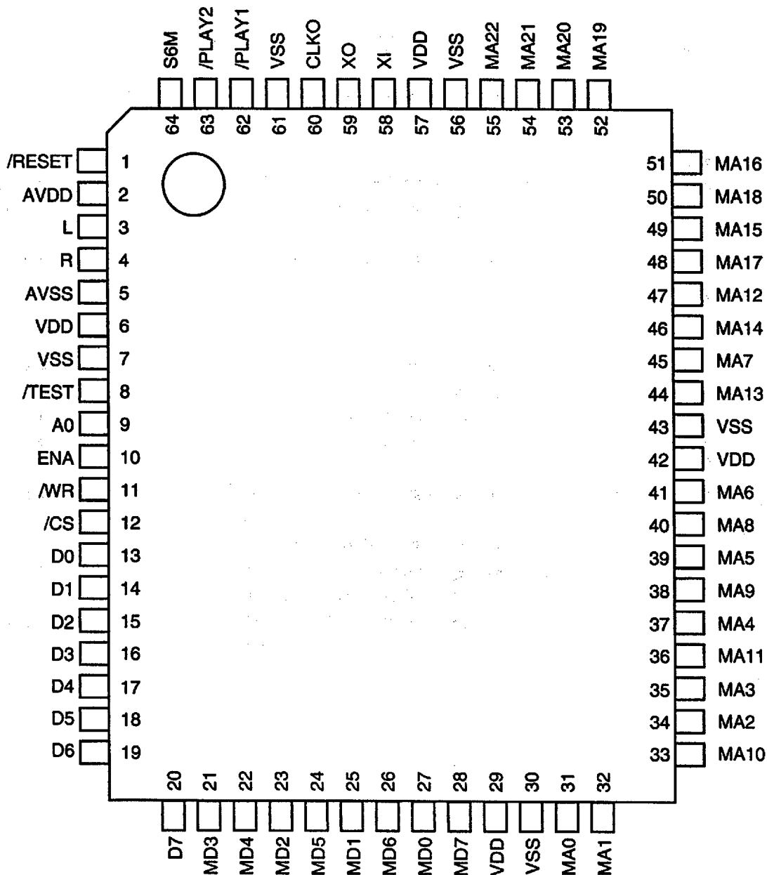
<64pin QFP Top View>
