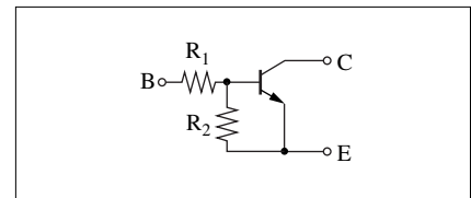
内部接続図
