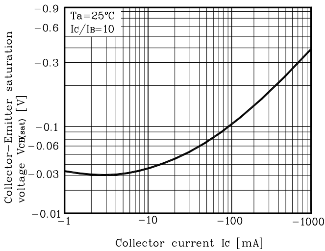
Fig. 3 V_{CE(sat)} - I_C
