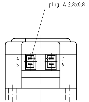
Seitenansicht von rechts
