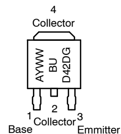
DPAK CASE 369C STYLE 1
