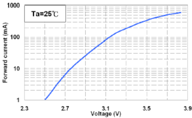
I_F - V_F
