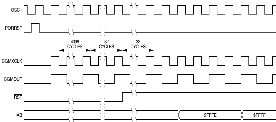
Figure 15-7. POR Recovery
