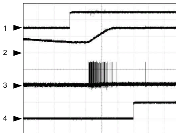
Non-Zero VDDQ S5 Enable
