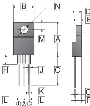
ITO-220
