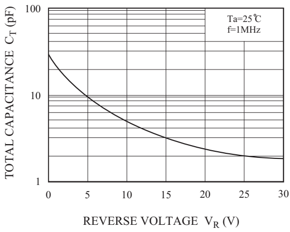
C_T - V_R
