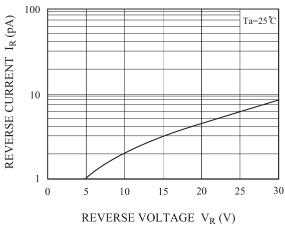
I_R - V_R
