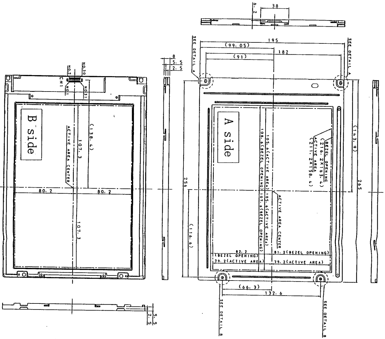
Fig 1 LQ10D34G OUTLINE DIMENSIONS
