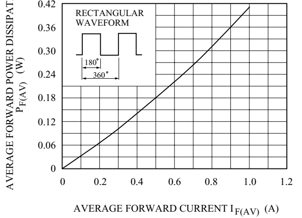
P_{F(AV)} - I_{F(AV)}
