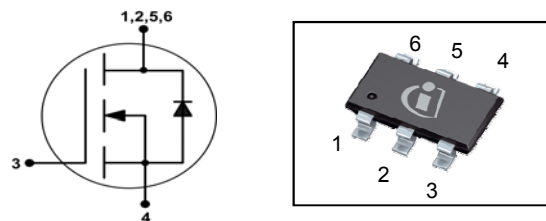
TSOP6
