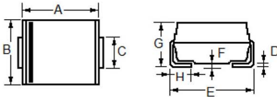
SMA (DO-214AC)
