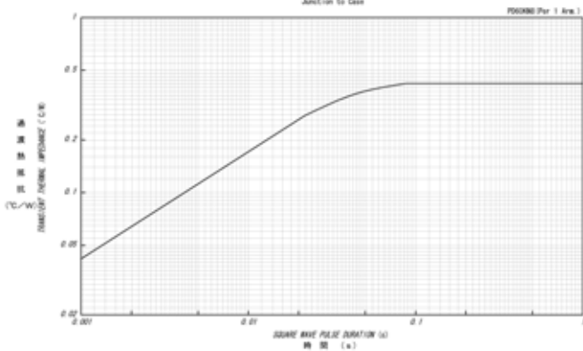
過渡熱抵抗特性 RULING TRANSIENT THERMAL IMPEDANCE
